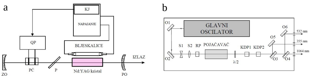
Слика 3.7: Панел а: Схема рада главног осцилатора ласерског система Ekspla NL-311-SH-TH. Панел б: Приказ распореда оптичких компонената ласерског система Ekspla NL-311-SH-TH. Слике са оба панела су преузете из [69], а модификоване су и преузете из [72].
