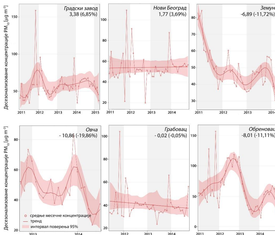
Слика 6.3.1.2. Тренд анализа масених концентрација PM_{10} са процењеном стопом промене током анализираниог периода на шест мерних места у Београду
