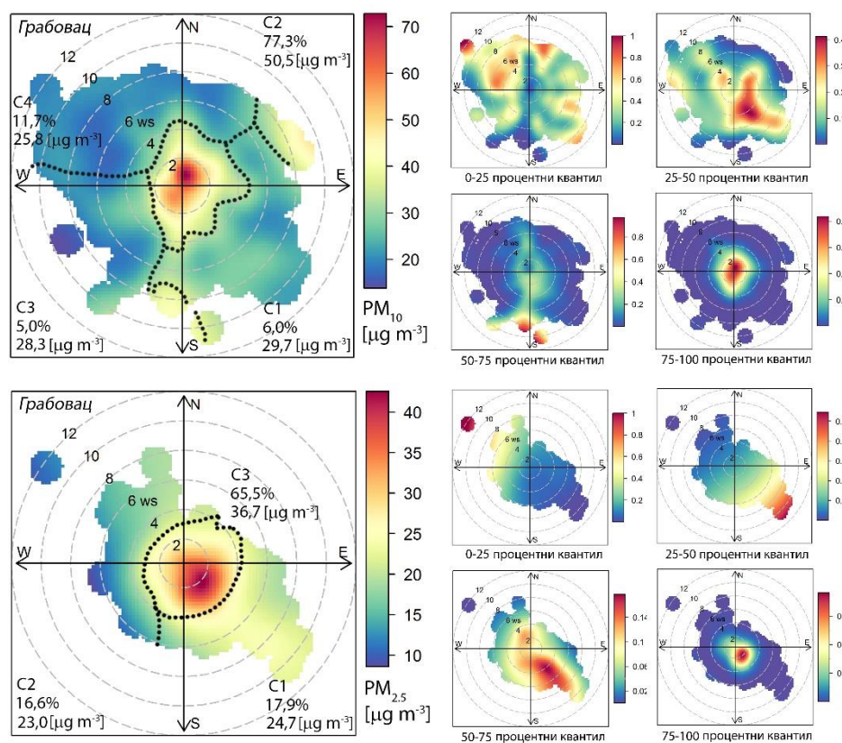
Слика 6.3.3.4. Зависност масених концентрација PM_{10} (слика горе) и PM_{2.5} (слика доле) од правца и брзине ветра ( ws [m s -1 ]) и поларна кластер анализа (лево), и анализа у четири опсега процентних квантила функцијом условне вероватноће (CBPF) (десно); мерно место Грабовац у периоду од 2011. до 2014. године
