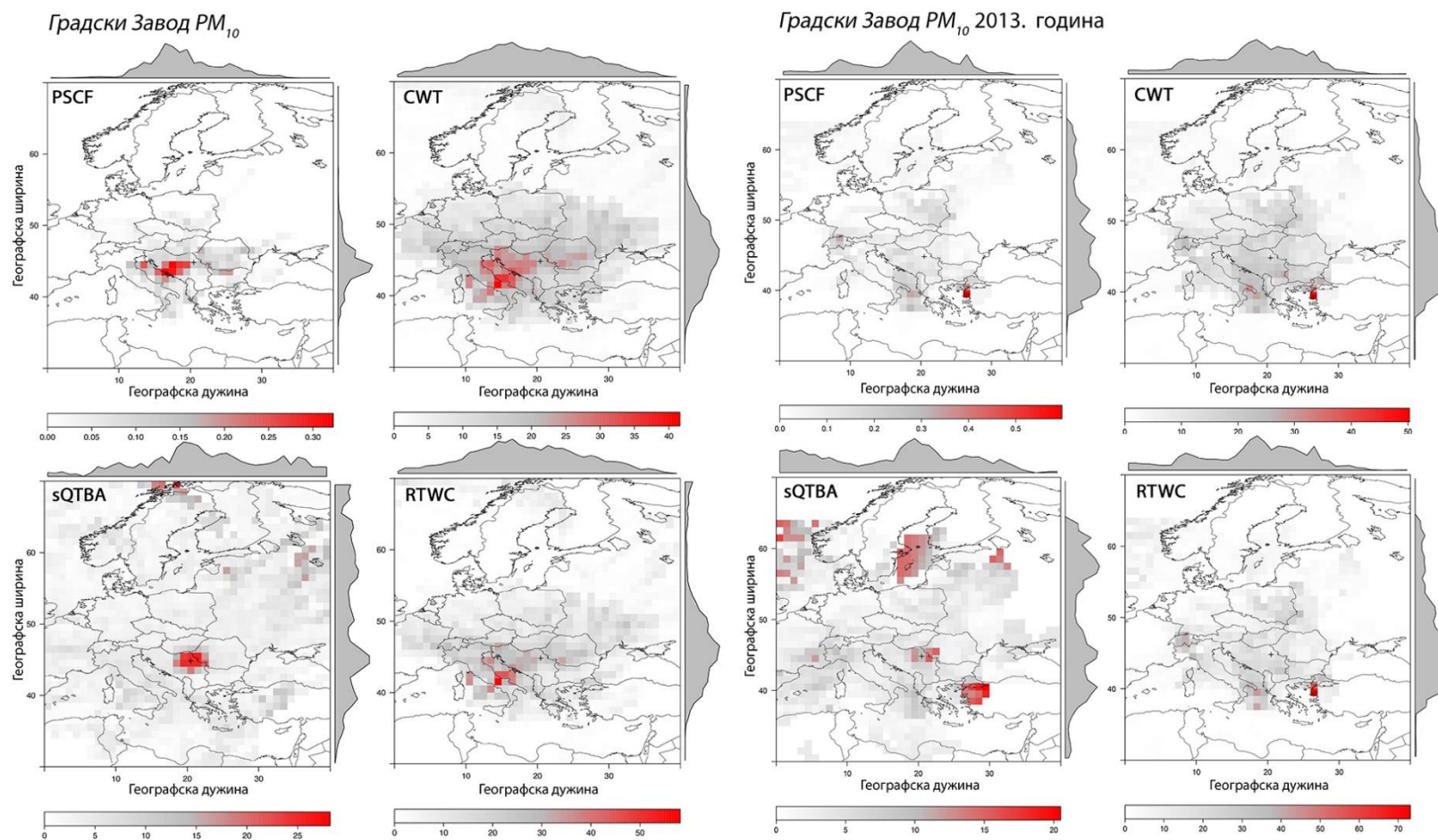
Слика Д-4. Резултати примене хибридних рецепторских модела PSCF (вероватноћа), CWT , sQTBA и RTWC [ \mu g\ m^{-3} ] за анализу транспорта PM_{10} на мерном месту Градски завод у различитим периодима
