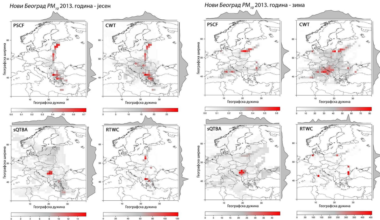
Слика Д-9. Резултати примене хибридних рецепторских модела PSCF (вероватноћа), CWT , sQTBA и RTWC [ \mu g\ m^{-3} ] за анализу транспорта PM_{10} на мерном месту Нови Београд у различитим периодима
