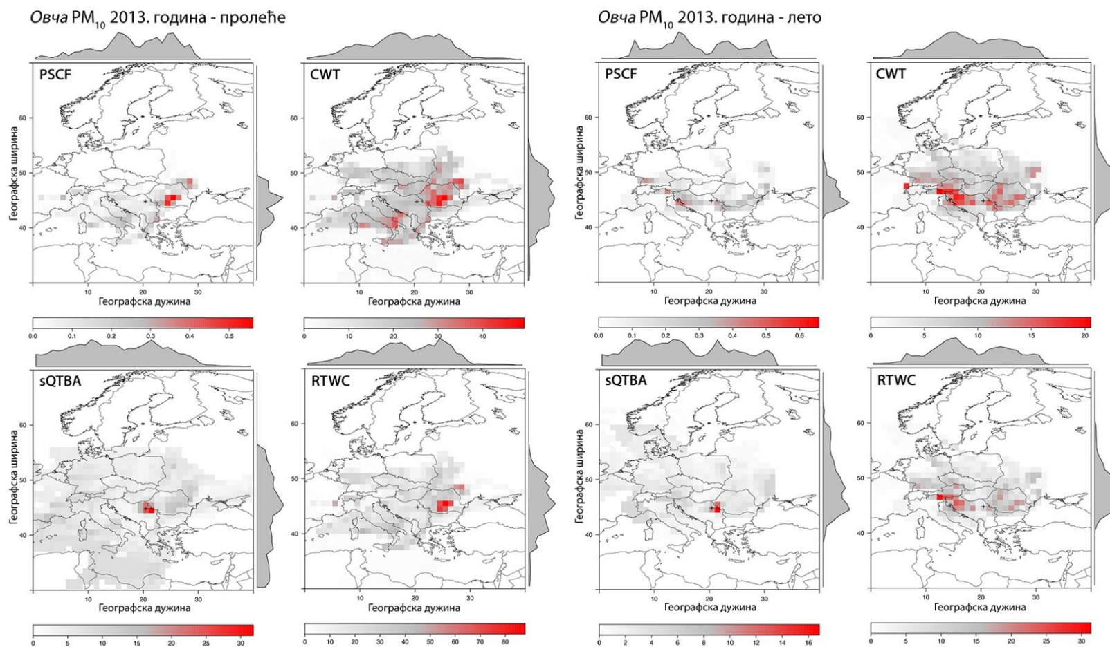
Слика Д-14. Резултати примене хибридних рецепторских модела PSCF (вероватноћа), CWT , sQTBA и RTWC [ \mu g m^{-3} ] за анализу транспорта PM_{10} на мерном месту Овча у различитим периодима
