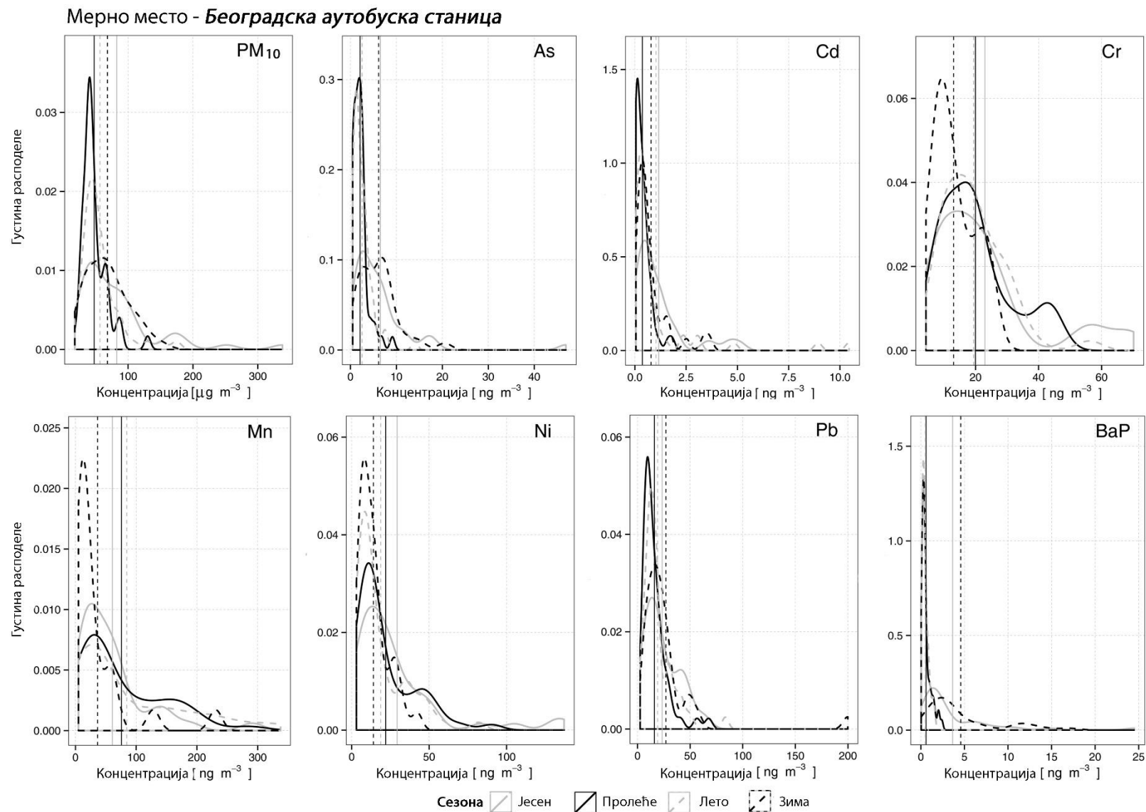
Слика Б-4. Функција густине расподеле концентрација PM 10 , As, Cd, Cr, Mn, Ni, Pb и BaP на мерном месту Београдска аутобуска станица за период од 2011. до 2015. године
