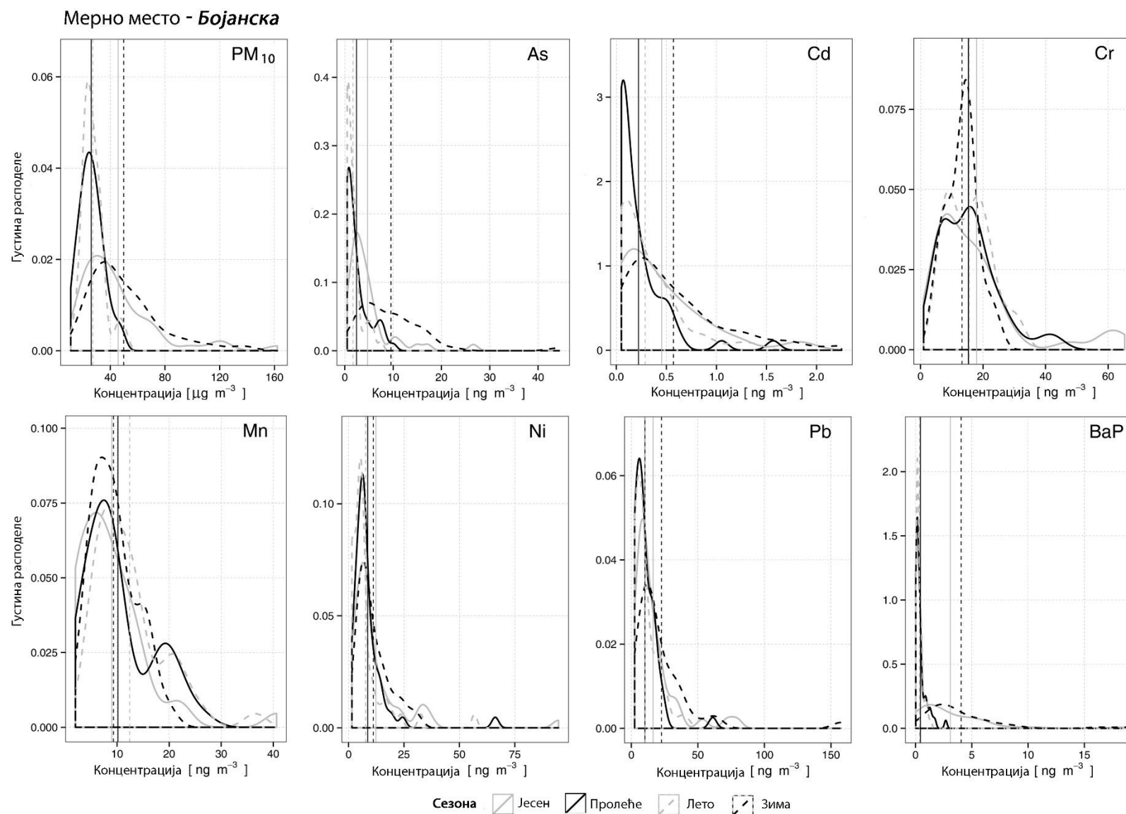
Слика Б-3. Функција густине расподеле концентрација PM 10 , As, Cd, Cr, Mn, Ni, Pb и BaP на мерном месту Бојанска за период од 2011. до 2015. године
