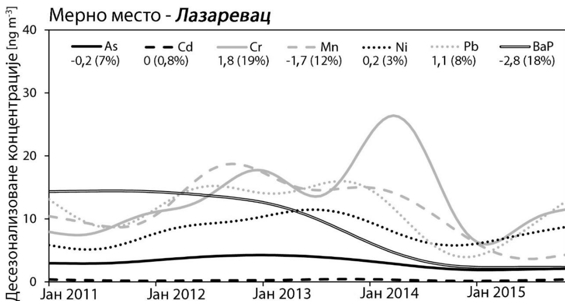
Слика В-13. Тренда анализа концентрација As, Cd, Cr, Mn, Ni, Pb и B[a]P [ \text{ng m}^{-3} ] са стопом промене на мерном месту Лазаревац за период од 2011. до 2015. године
