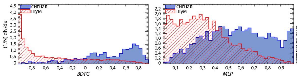
Слика 6.4.1.2. Резултати MVA класификационих метода за PM_{10} класификациону вредност 100 \mu g m^{-3} (лево) и 50 \mu g m^{-3} (десно) за мерно место Градски завод
