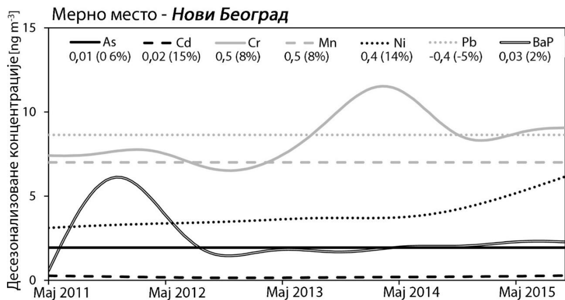
Слика В-7. Тренда анализа концентрација As, Cd, Cr, Mn, Ni, Pb и B[a]P [ \text{ng m}^{-3} ] са стопом промене на мерном месту Нови Београд за период од 2011. до 2015. године
