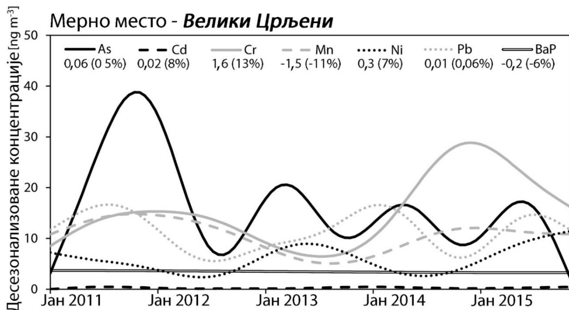
Слика В-15. Тренда анализа концентрација As, Cd, Cr, Mn, Ni, Pb и B[a]P [ng m -3 ] са стопом промене на мерном месту Велики Црљени за период од 2011. до 2015. године
