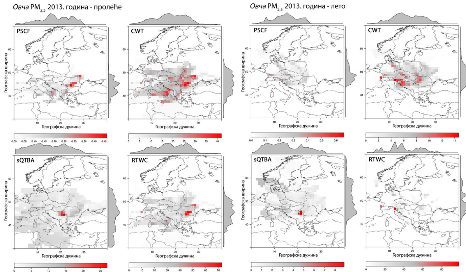
Слика Д-17. Резултати примене хибридних рецепторских модела PSCF (вероватноћа), CWT , sQTBA и RTWC [ \mu g\ m^{-3} ] за анализу транспорта PM_{2.5} на мерном месту Овча у различитим периодима
