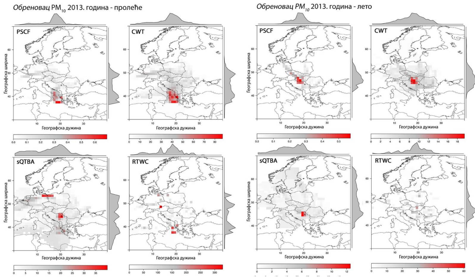
Слика Д-12. Резултати примене хибридних рецепторских модела PSCF (вероватноћа), CWT , sQTBA и RTWC [ \mu g\ m^{-3} ] за анализу транспорта PM_{10} на мерном месту Обреновац у различитим периодима
