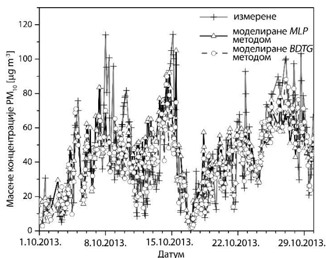
Слика 6.4.2.1. Поређење временске серије измерених и моделираних PM_{10} концентрација [ \mu g m^{-3} ] на мерном месту Грабовац
