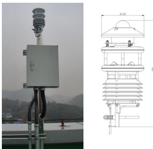
Слика 4.6.1. Спољашњи изглед метеоролошке станице (лево), и приказ главе са сензорима (десно)
