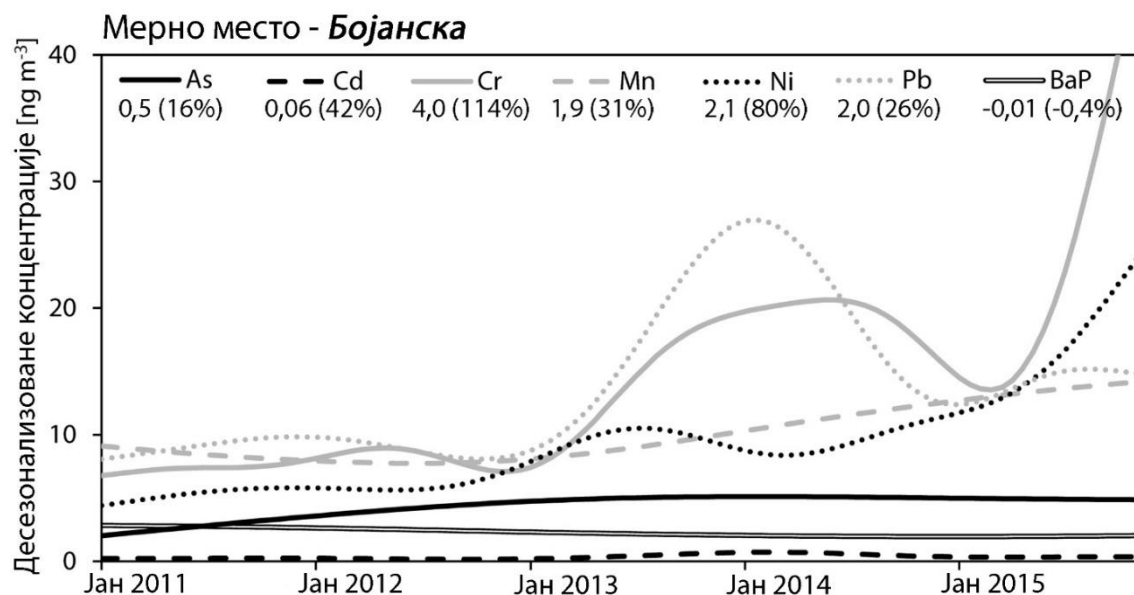
Слика В-3. Тренда анализа концентрација As, Cd, Cr, Mn, Ni, Pb и B[a]P [ \text{ng m}^{-3} ] са стопом промене на мерном месту Бојанска за период од 2011. до 2015. године
