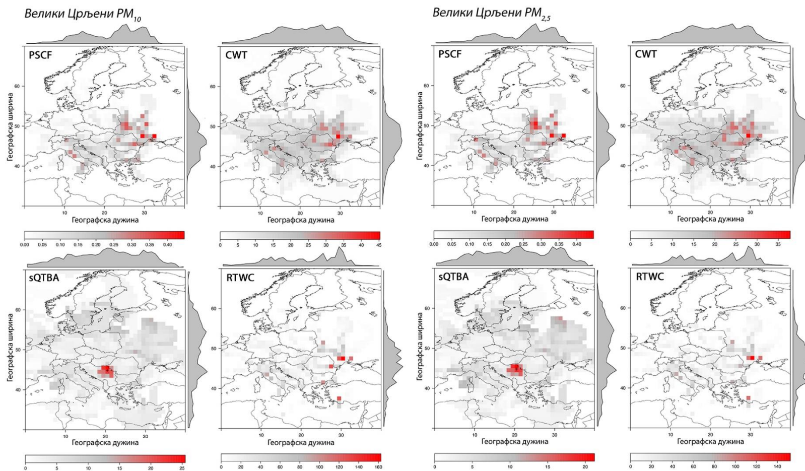
Слика Д-19. Резултати примене хибридних рецепторских модела PSCF (вероватноћа), CWT , sQTBA и RTWC [ \mu\text{g m}^{-3} ] за анализу транспорта \text{PM}_{10} и \text{PM}_{2,5} на мерном месту Велики Црљени у различитим периодима
