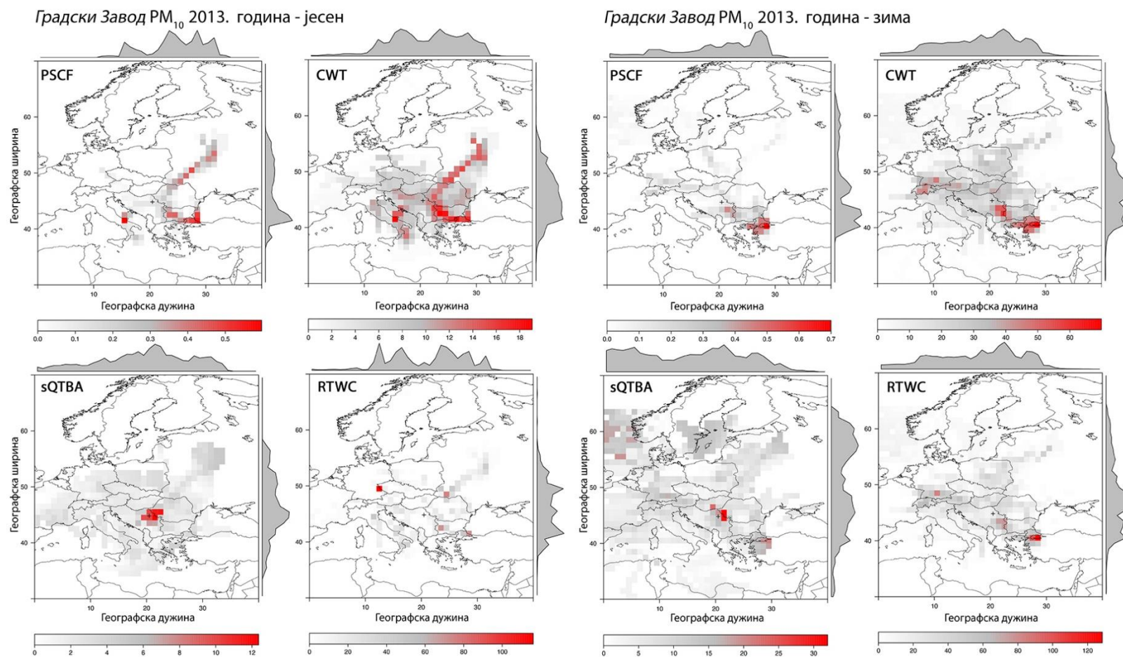
Слика Д-6. Резултати примене хибридних рецепторских модела PSCF (вероватноћа), CWT , sQTBA и RTWC [ \mu g\ m^{-3} ] за анализу транспорта PM_{10} на мерном месту Градски завод у различитим периодима
