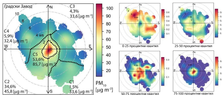
Слика 6.3.3.1. Зависност масених концентрација PM_{10} од правца и брзине ветра ( ws [m s^{-1}] ) и поларна кластер анализа (лево), и анализа у четири опсега процентних квантила функцијом условне вероватноће ( CBPF ) (десно); мерно место Градски завод од 2011. до 2015. године
