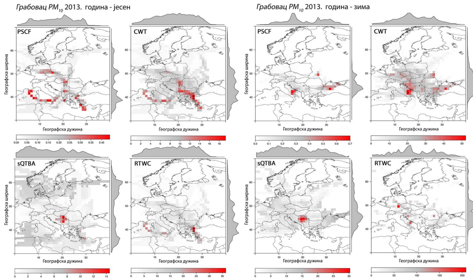
Слика Д-3. Резултати примене хибридних рецепторских модела PSCF (вероватноћа), CWT , sQTBA и RTWC [ \mu\text{g m}^{-3} ] за анализу транспорта PM_{10} на мерном месту Грабовац у различитим периодима
