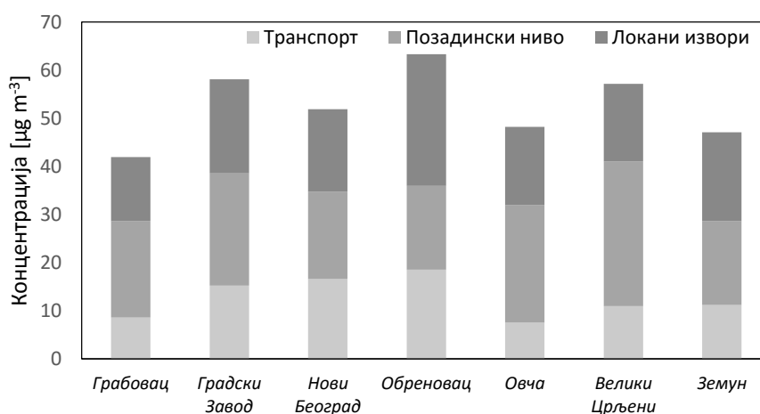
Слика 6.3.4.1.1. Удео транспорта, позадинског нивоа и локалних извора измереним концентрацијама PM_{10} на седам мерних места у Београду у периоду од 2011. до 2015. године добијен применом TSA
