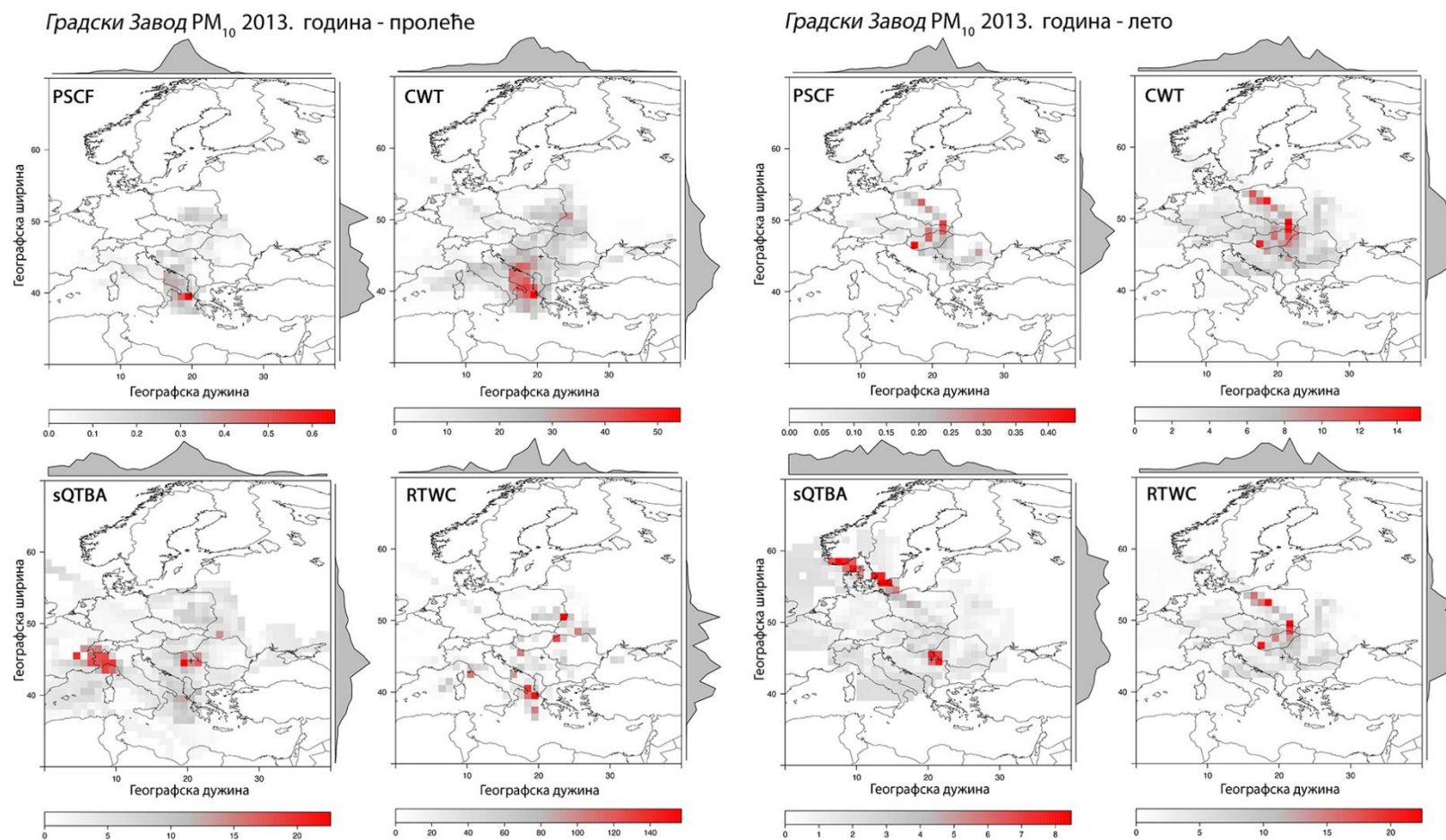
Слика Д-5. Резултати примене хибридних рецепторских модела PSCF (вероватноћа), CWT , sQTBA и RTWC [ \mu g\ m^{-3} ] за анализу транспорта PM_{10} на мерном месту Градски завод у различитим периодима
