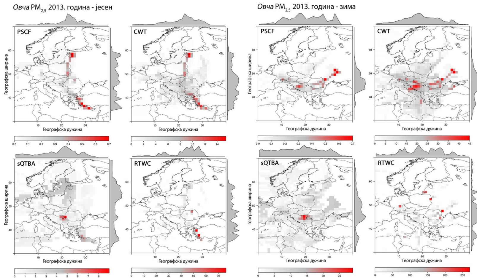
Слика Д-18. Резултати примене хибридних рецепторских модела PSCF (вероватноћа), CWT , sQTBA и RTWC [ \mu\text{g m}^{-3} ] за анализу транспорта PM_{2,5} на мерном месту Овча у различитим периодима
