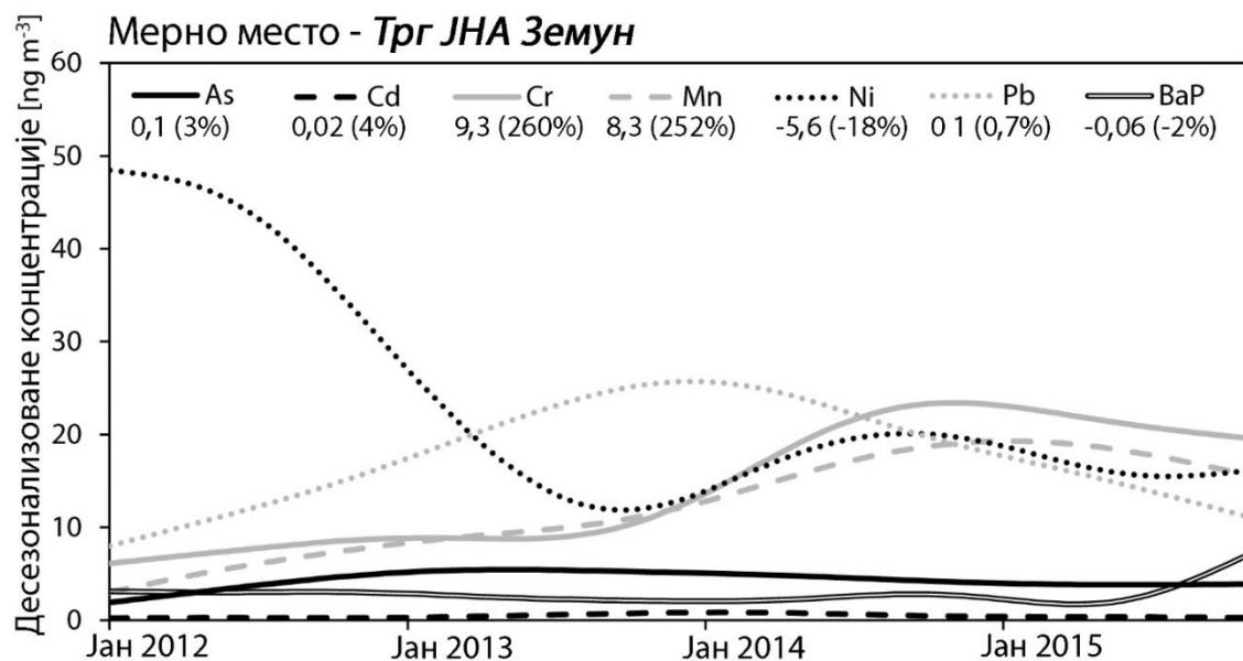
Слика В-8. Тренда анализа концентрација As, Cd, Cr, Mn, Ni, Pb и B[a]P [ \text{ng m}^{-3} ] са стопом промене на мерном месту Трг ЈНА Земун за период од 2012. до 2015. године
