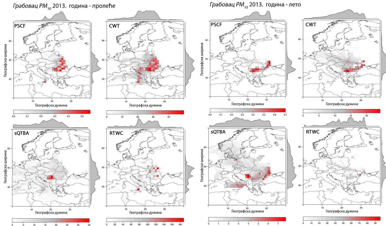
Слика Д-2. Резултати примене хибридних рецепторских модела PSCF (вероватноћа), CWT , sQTBA и RTWC [ \mu\text{g m}^{-3} ] за анализу транспорта PM_{10} на мерном месту Грабовац у различитим периодима
