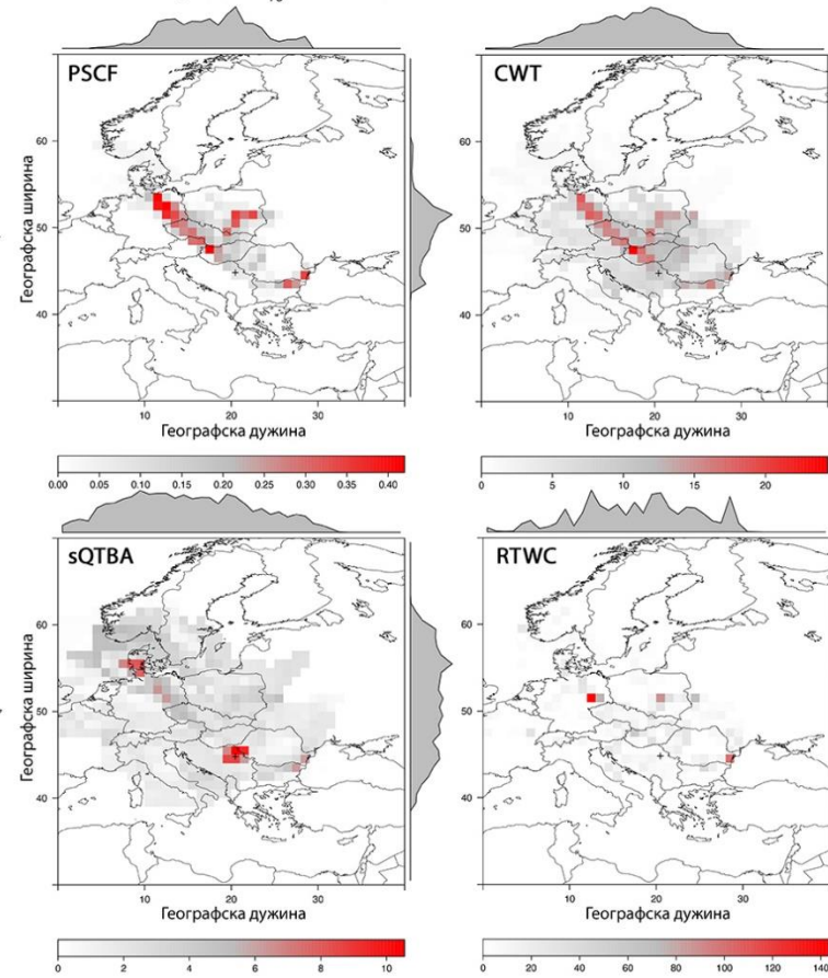
Нови Београд PM_{10} 2013. година - лето
