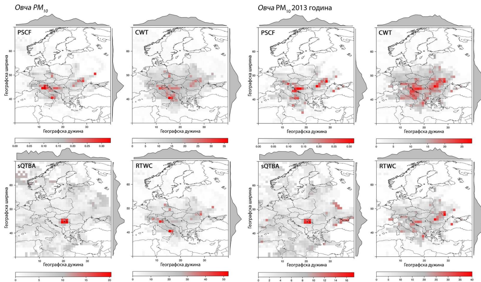
Слика Д-13. Резултати примене хибридних рецепторских модела PSCF (вероватноћа), CWT , sQTBA и RTWC [ \mu g m^{-3} ] за анализу транспорта PM_{10} на мерном месту Овча у различитим периодима
