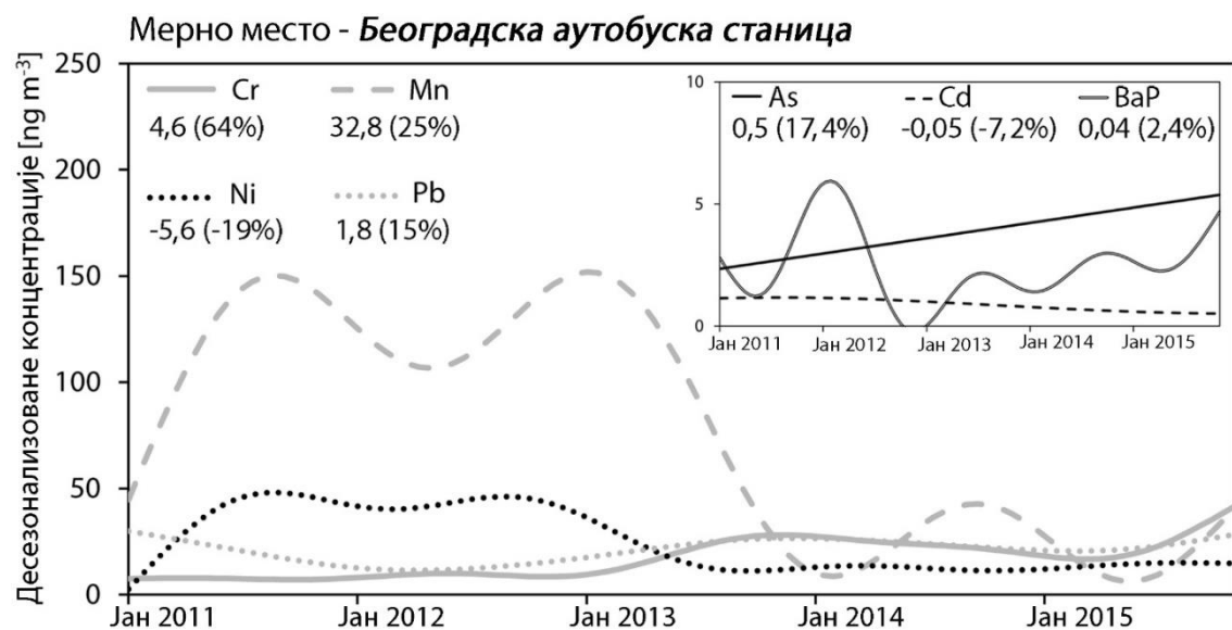
Слика В-4. Тренда анализа концентрација As, Cd, Cr, Mn, Ni, Pb и B[a]P [ \text{ng m}^{-3} ] са стопом промене на мерном месту Београдска аутобуска станица за период од 2011. до 2015. године
