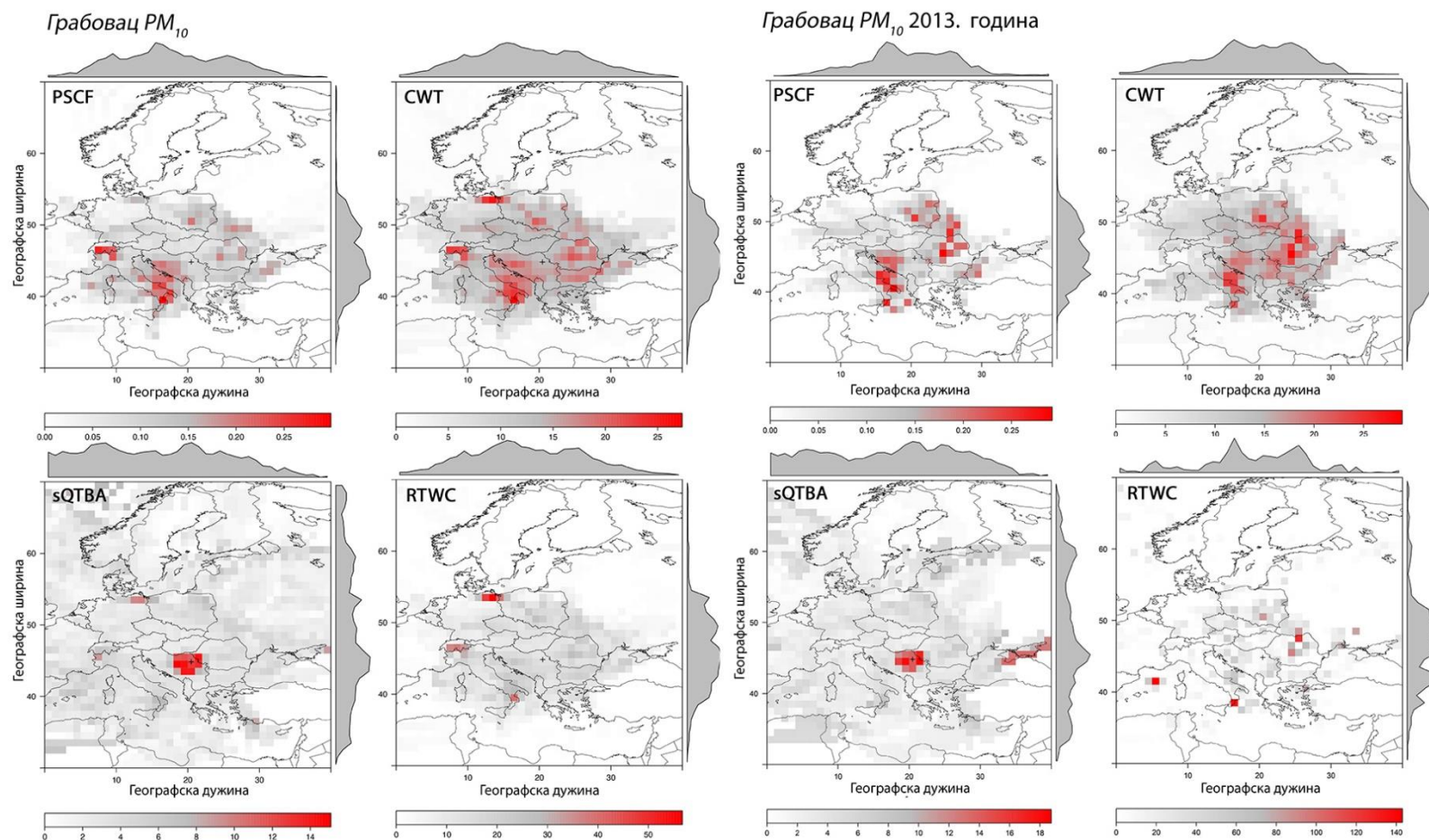
Слика Д-1. Резултати примене хибридних рецепторских модела PSCF (вероватноћа), CWT , sQTBA и RTWC [ \mu g\ m^{-3} ] за анализу транспорта PM_{10} на мерном месту Грабовац у различитим периодима
