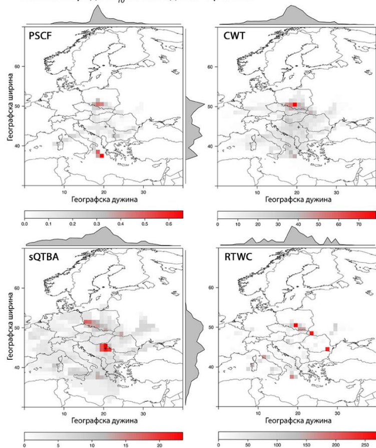
Нови Београд PM_{10} 2013. година - пролеће
