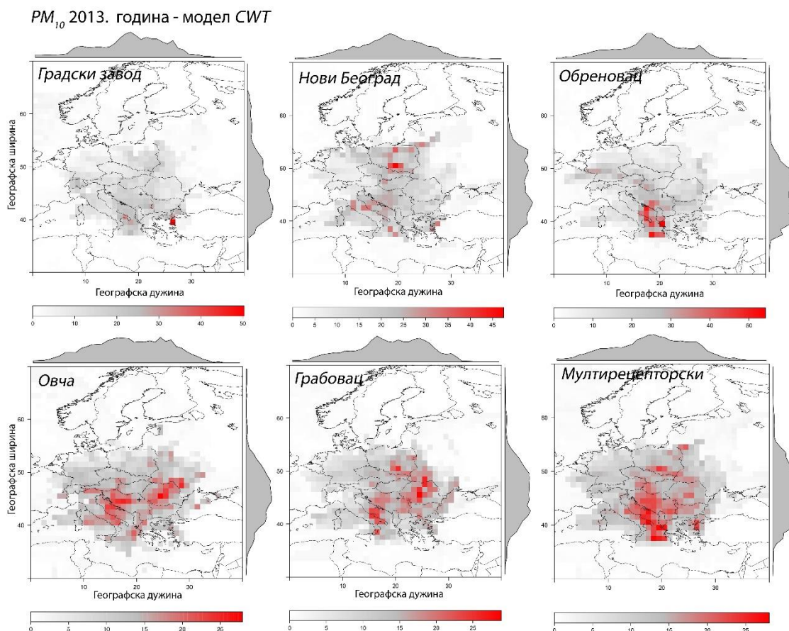
Слика 6.3.4.3.9. Резултати примене хибридног рецепторског модела CWT и његове мултирецепторске варијанте [ \mu\text{g m}^{-3} ] у анализи транспорта PM_{10} на пет мерних места у Београду током 2013. године
