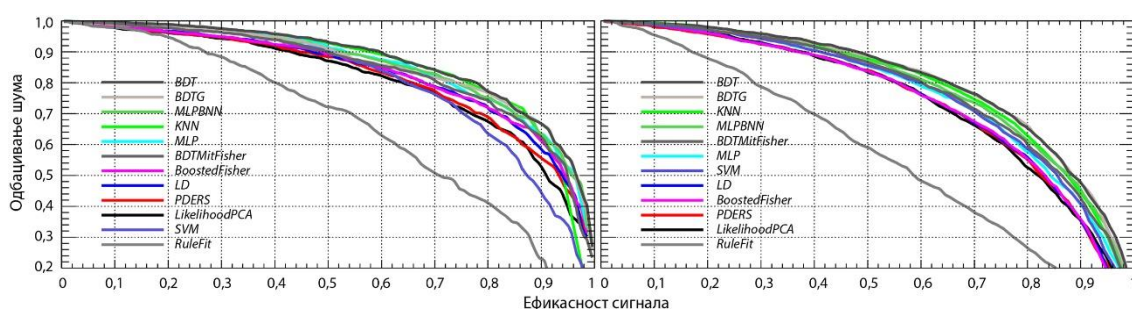
Слика 6.4.1.1. ROC крива за MVA класификационе методе са PM_{10} нивоом за класификацију од 100 \mu g m^{-3} (лево) и 50 \mu g m^{-3} (десно) на свим мерним местима
