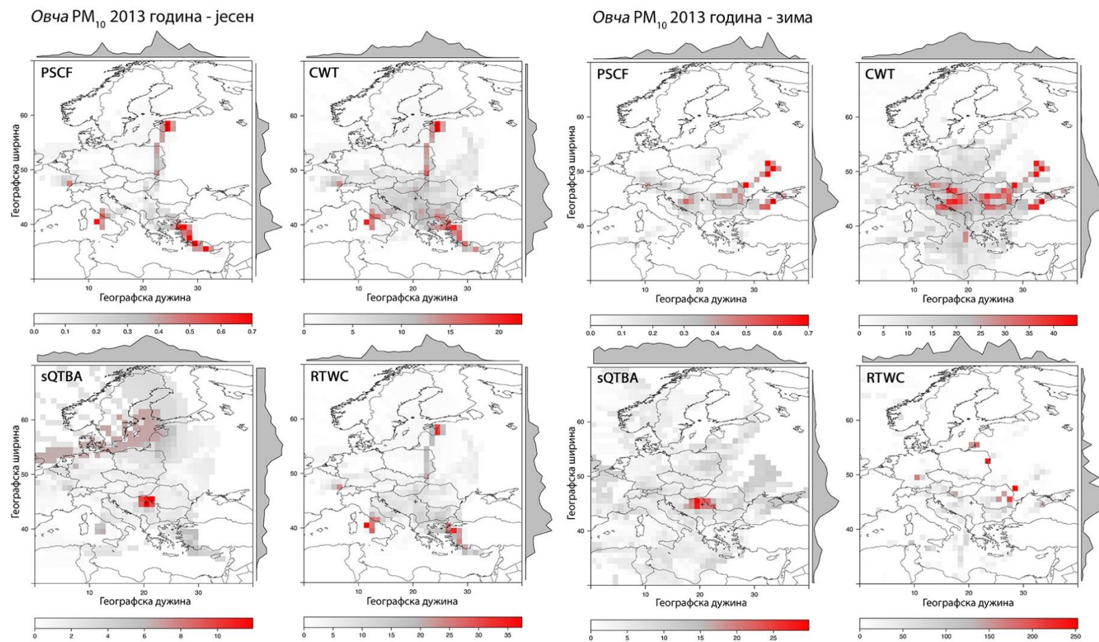
Слика Д-15. Резултати примене хибридних рецепторских модела PSCF (вероватноћа), CWT , sQTBA и RTWC [ \mu\text{g m}^{-3} ] за анализу транспорта PM 10 на мерном месту Овча у различитим периодима
