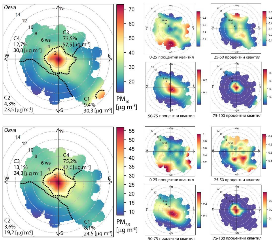
Слика 6.3.3.5. Зависност масених концентрација PM_{10} (слика горе) и PM_{2.5} (слика доле) од правца и брзине ветра (ws [m s -1 ]) и поларна кластер анализа (лево), и анализа у четири опсега процентних квантила функцијом условне вероватноће (CBPF) (десно); мерно место Овча у периоду од 2012. до 2014. године
