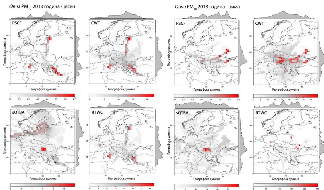
Слика 6.3.4.3.7. Резултати примене хибридних рецепторских модела PSCF (вероватноћа), CWT , sQTBA и RTWC [ \mu g m^{-3} ] у анализи транспорта PM_{10} на мерном месту Овча током јесени (лево) и зиме 2013. године (десно)
